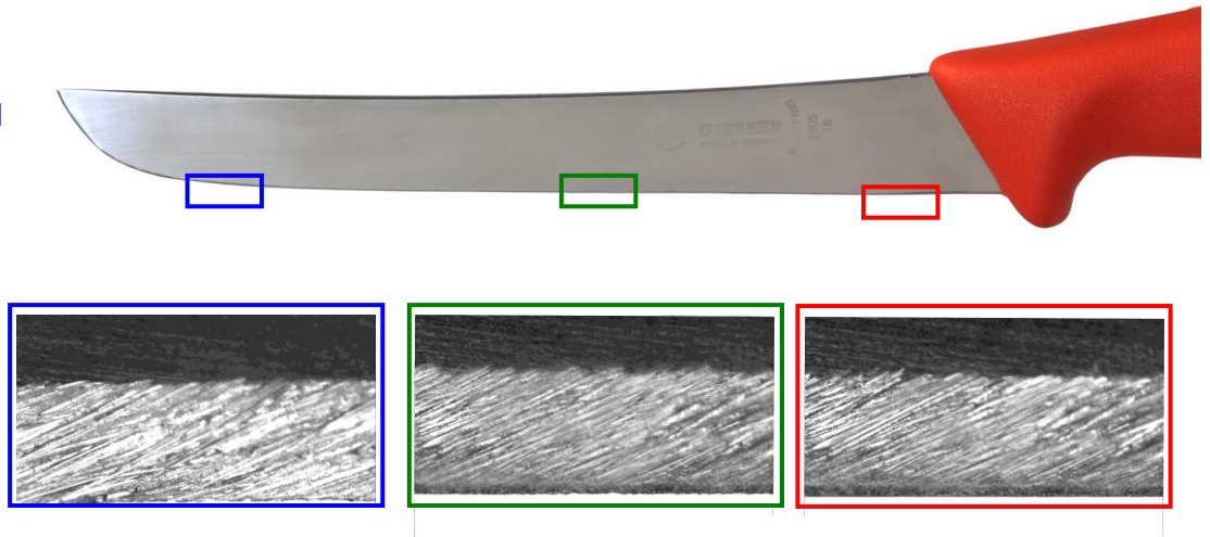
Konvexes Schleifen
